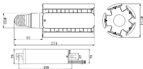
400形相当(電源別置タイプ)
