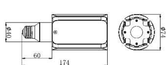
100形相当(電源内蔵タイプ)
