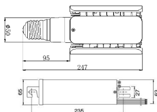
250形相当(電源別置タイプ)
