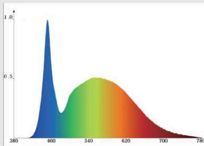
一般的な LED の分光分布
