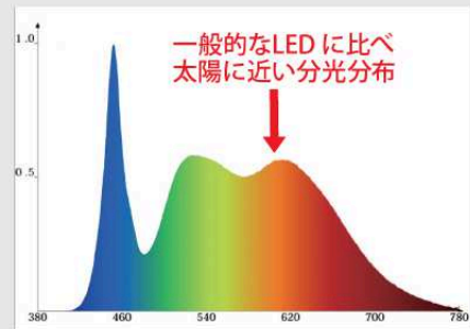
太陽に近い分光分布で色再現性が高い
