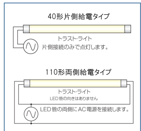
結線図
